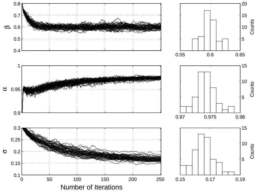
FIG. 2.2 – Trajectoires des paramètres estimés par Monte Carlo EM en utilisant l'estimateur \hat{\gamma}_n^m (modèle de volatilité stochastique, 5000 observations) [Olsson et al., 2006b].
