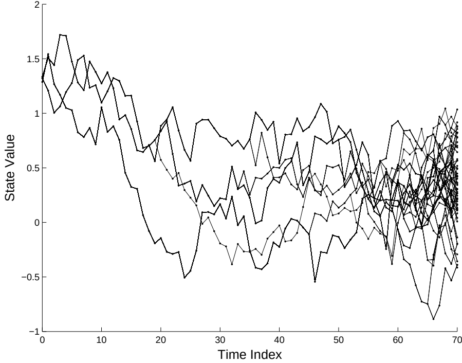
FIG. 2.1 – Trajectoires des particules pour n = 70 et N = 50 (modèle de volatilité stochastique) [Cappé et al., 2005].
