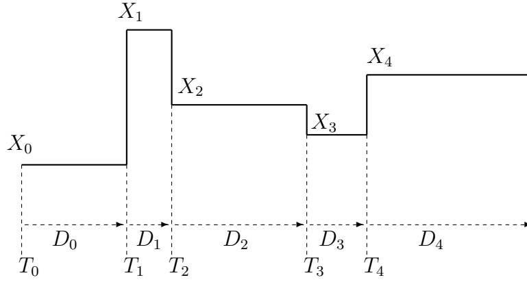
FIG. 3.1 – Principe de l'algorithme de simulation à temps continu [Cappé et al., 2003].
