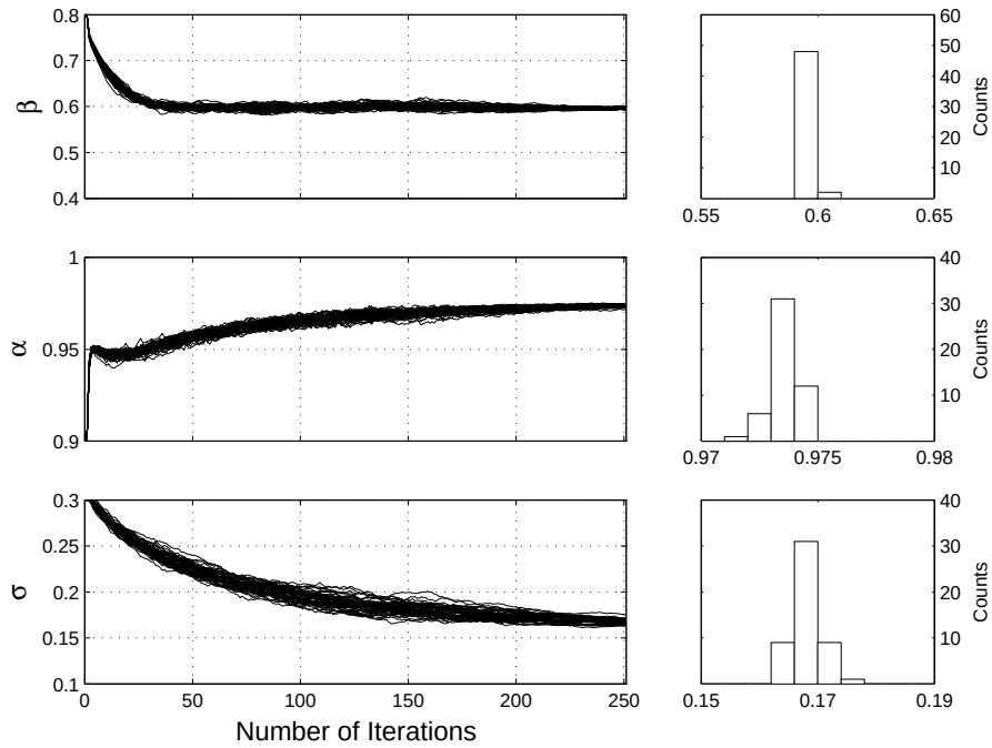
FIG. 2.3 – Trajectoires des paramètres estimés par Monte Carlo EM en utilisant l'estimateur à délai fixe \hat{\gamma}_n^{m,\Delta} pour \Delta = 40 (même modèle, données et nombre de particules que pour la figure 2.2) [Olsson et al., 2006b].
