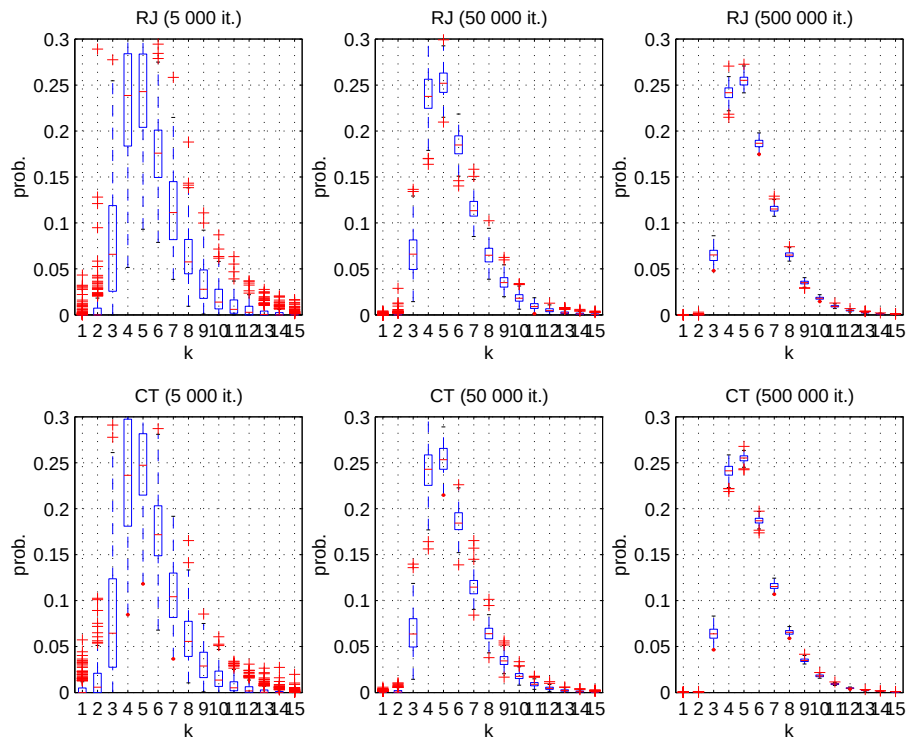
FIG. 3.2 – Estimation de la loi a posteriori du nombre de composantes dans un modèle de mélange de gaussiennes à nombre de composantes inconnues en utilisant l'algorithme MCMC à saut réversible (figures du haut — label « RJ ») ou l'algorithme à temps continu (en bas — label « CT »). Le nombre de simulations varie de, de gauche à droite, 5000 à 500000 itérations. Chaque figure résume 200 réalisations indépendantes sous forme de boxplots [Cappé et al., 2003].
